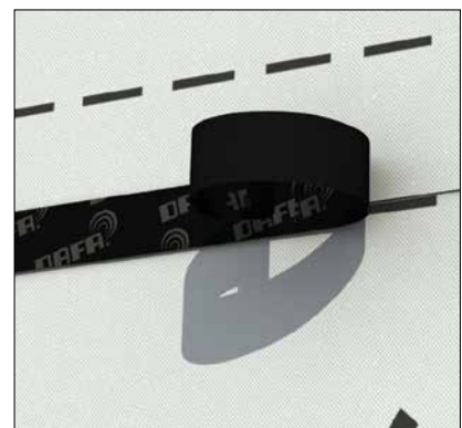
Her anvendes DAFA UV tape til overlap på DAFA Windfoil 95™ vindspærre
